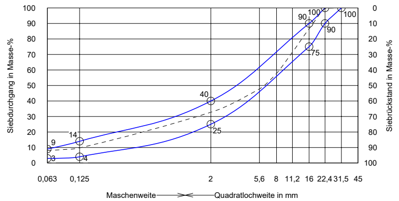
Sieblinienbereich für AC 22 T N
